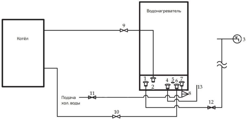
Рисунок 2. Подключение КЭВН
